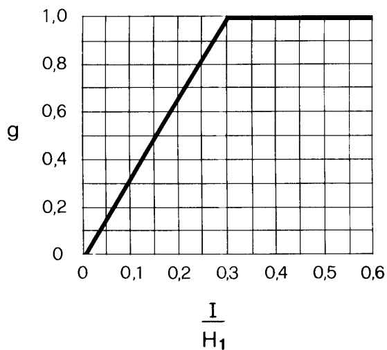
Diagramma 2: Determinazione del fattore di correzione g in zone edificate e boschive
