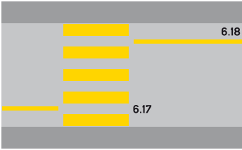
6.17 Passaggio pedonale 6.18 Linea vietante l'arresto (art. 77)
