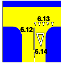
6.12 Ligne longitudinale continue 6.13 Ligne d'attente 6.14 Présignalisation de la ligne d'attente (art. 75)
