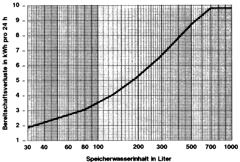
Diagramm 3: Bereitschaftsverluste für direkt befeuerte Speicherwasserwärmer mit atmosphärischen Gasbrenner
