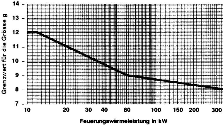
Diagramm 2: Grenzwert für die Grösse g für Heizkessel und Umlaufwärmeerzeuger mit atmosphärischen Gasbrennern
