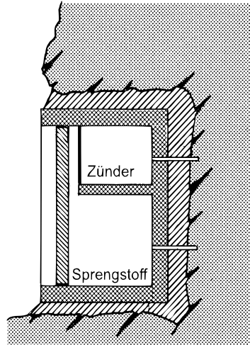
Querschnitt Hohlräume ausgemauert oder ausbetoniert
