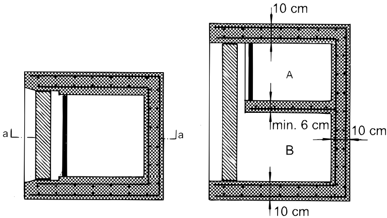
Schnitt a-a
